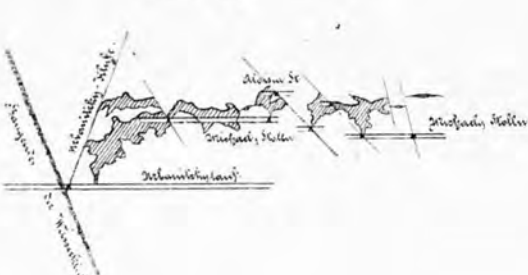
Diebedilthner Calmelagerstätte im Profil 1:4000 Fig. 3.
