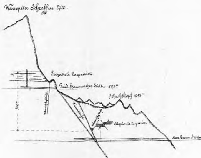
Profil durch Scherabstichkopf und Vampulter Schraffen und die Silberleithner Lagerstätte 1:30000. Fig 6.
