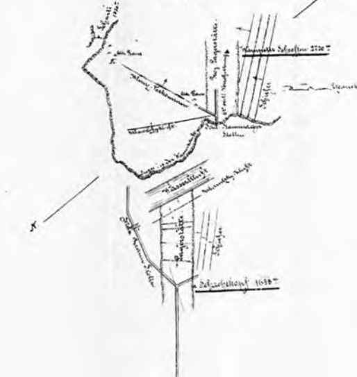
Grundriss der Silberleithner Lagerstätte. Fig. 11. 5 1:30000.
